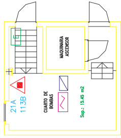
ÁTICO
